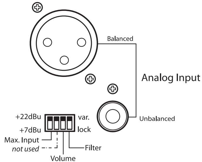
Rückseitige Anschlüsse & DIP-Schalter
